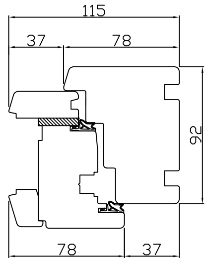
PRZEKRÓJ A-A
