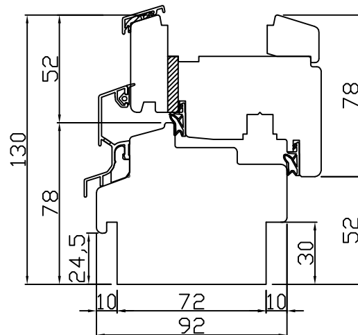
PRZEKRÓJ B-B
