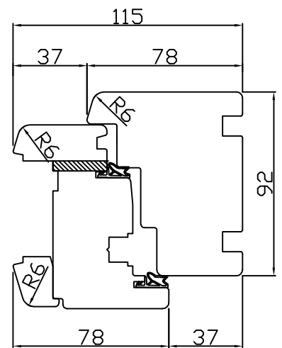
PRZEKRÓJ A-A
