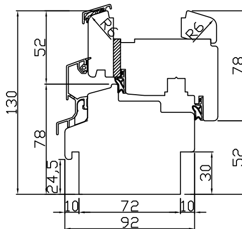
PRZEKRÓJ B-B
