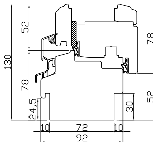
PRZEKRÓJ B-B
