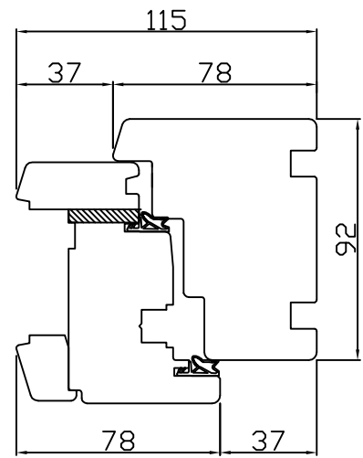
PRZEKRÓJ A-A
