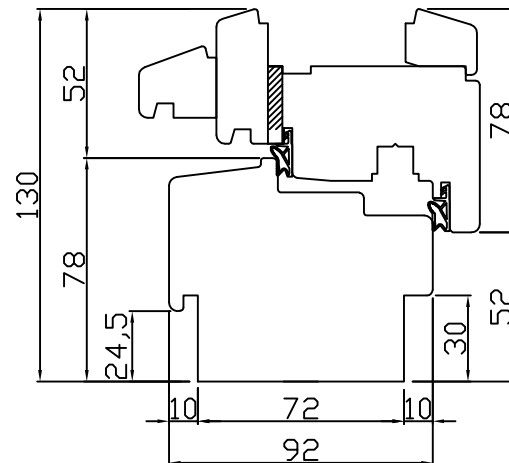
PRZEKRÓJ B-B
