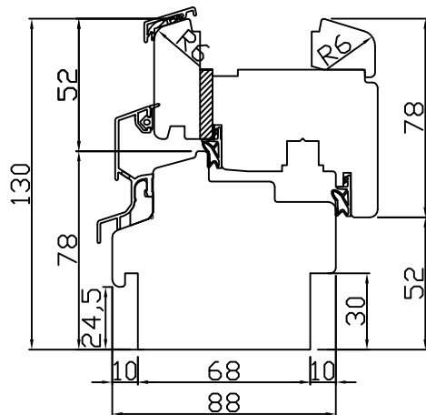
PRZEKRÓJ B-B
