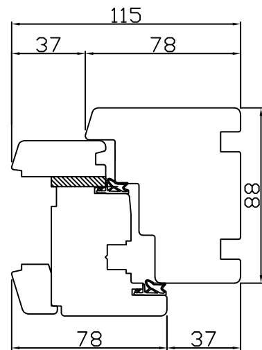
PRZEKRÓJ A-A
