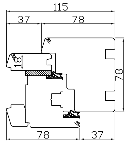
PRZEKRÓJ A-A
