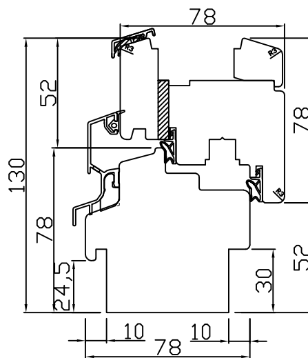
PRZEKRÓJ B-B
