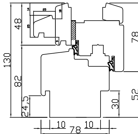
PRZEKRÓJ B-B
