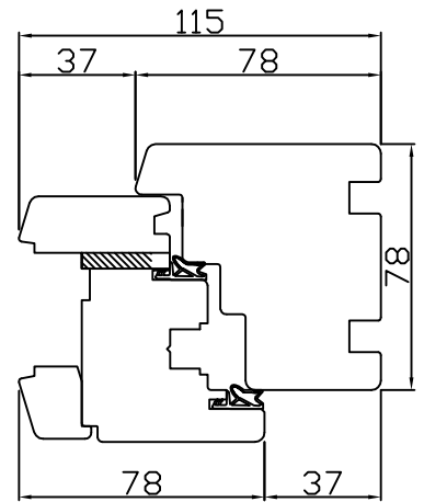
PRZEKRÓJ A-A
